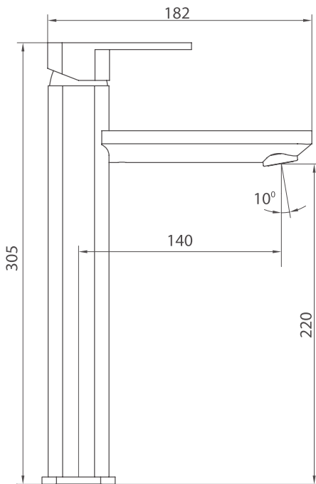
ברז רחצה גבוה 305444
